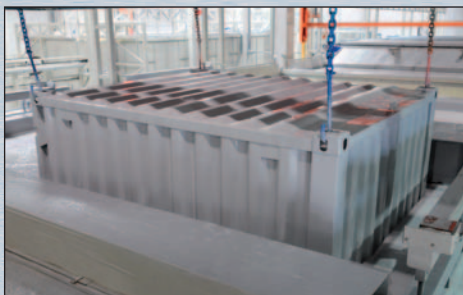
KTL -Grundierung im Tauchbecken
